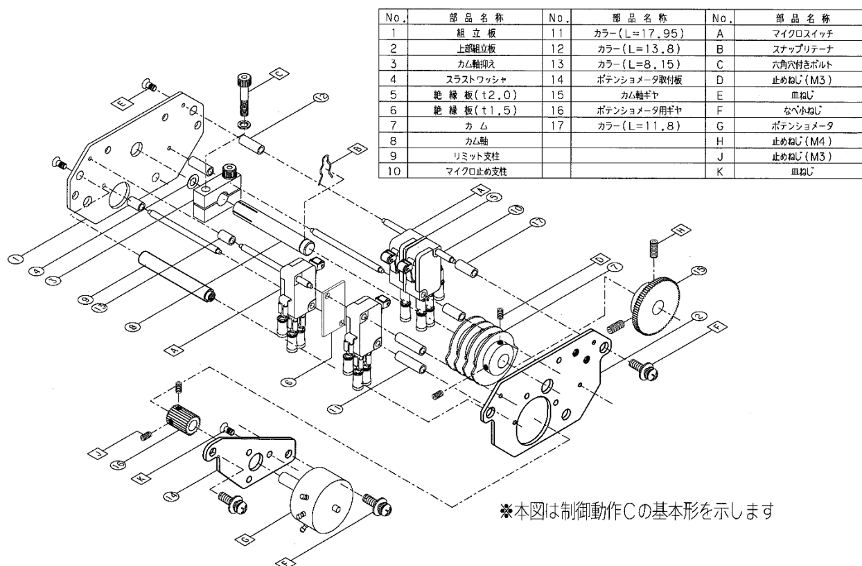
図 1 2 : スイッチ部の構造
