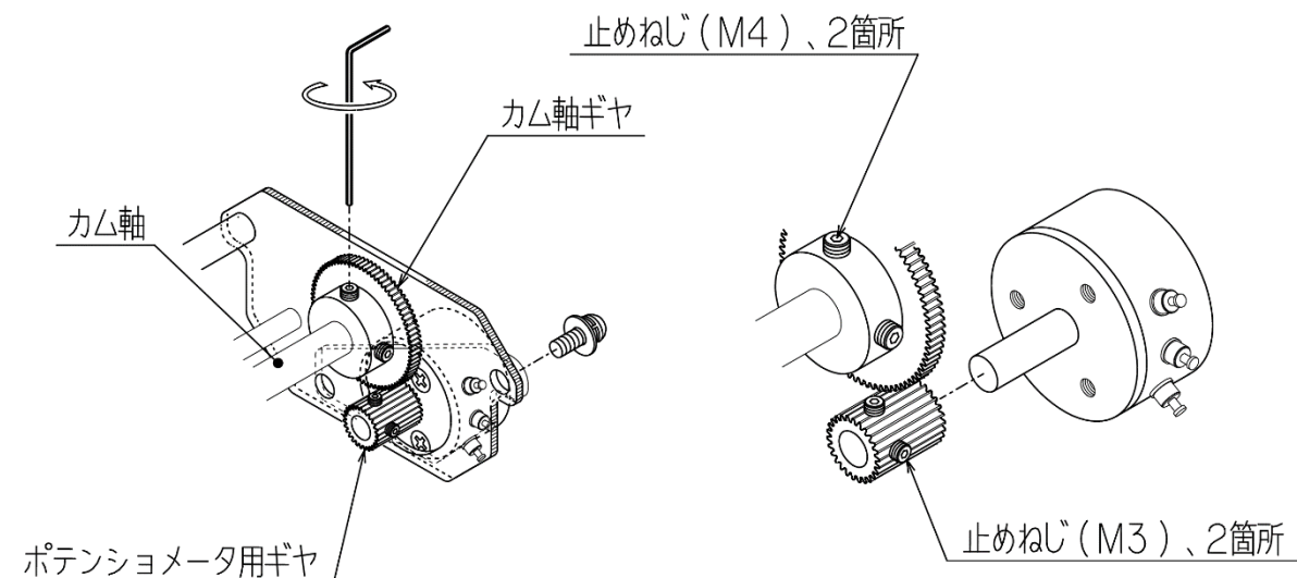
図 1 1 : ポテンショメータの調整
