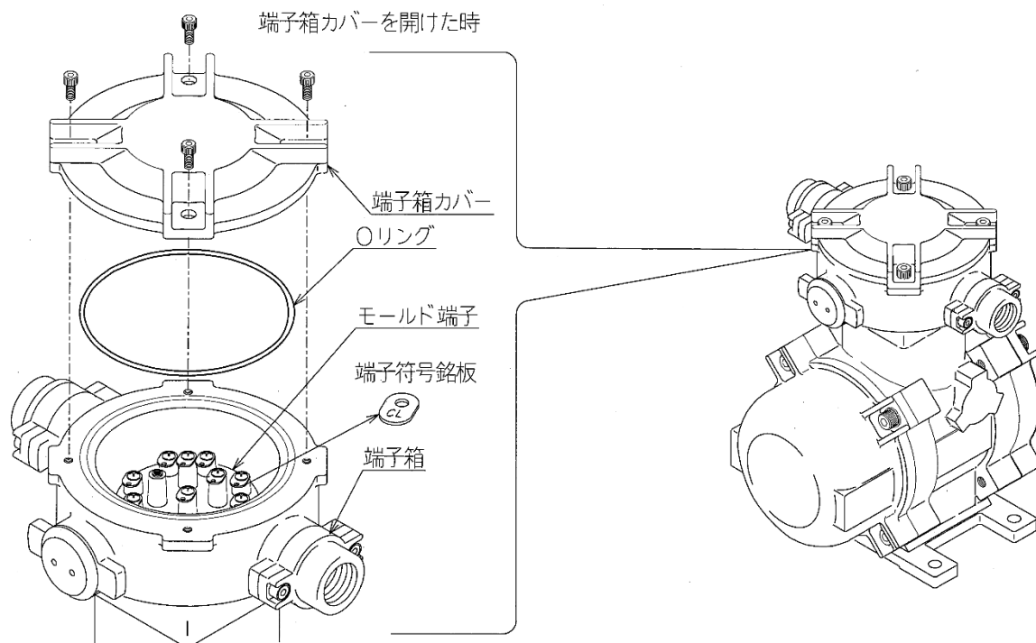
図4：配線準備
