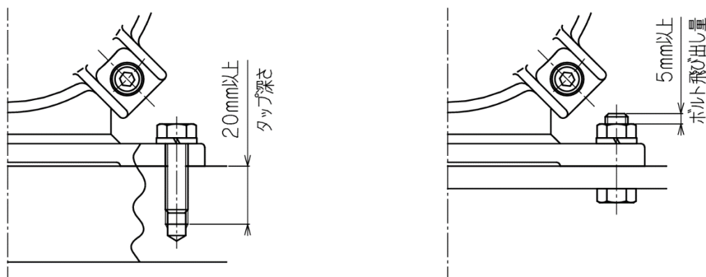
図 2 : 固定方法
