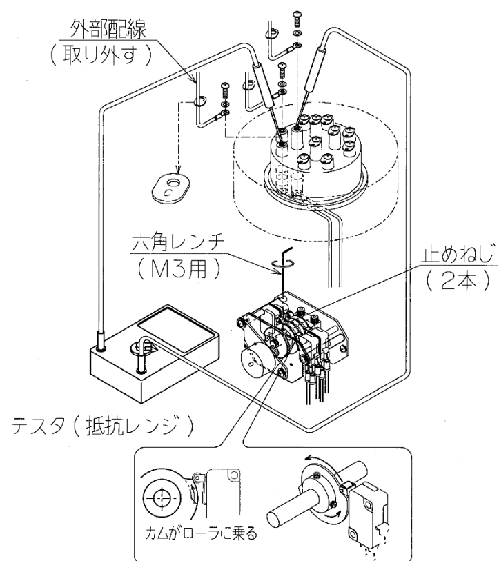
図9：スイッチ調整
