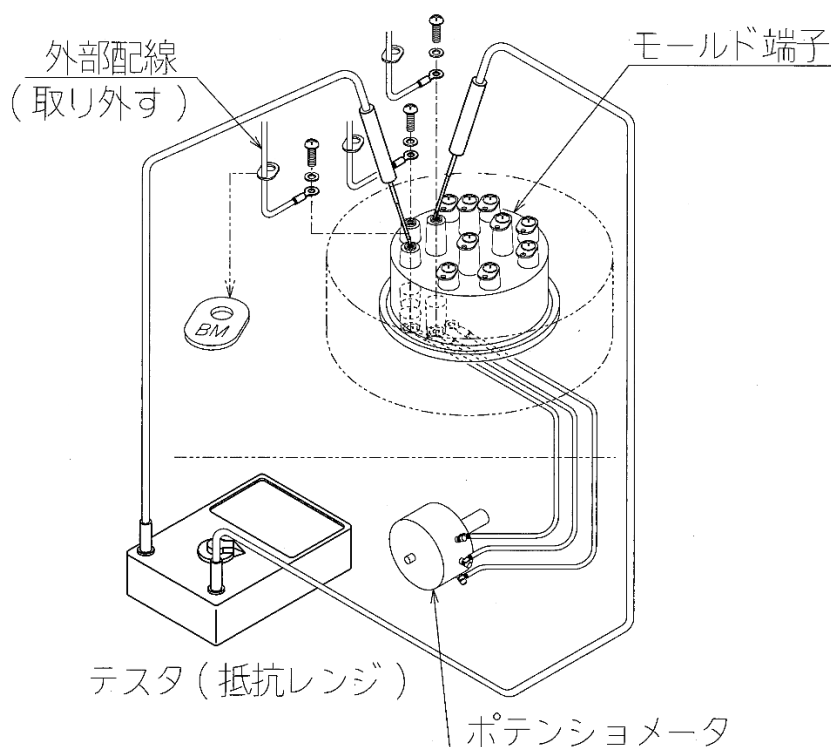
図8：ポテンシオメータの点検
