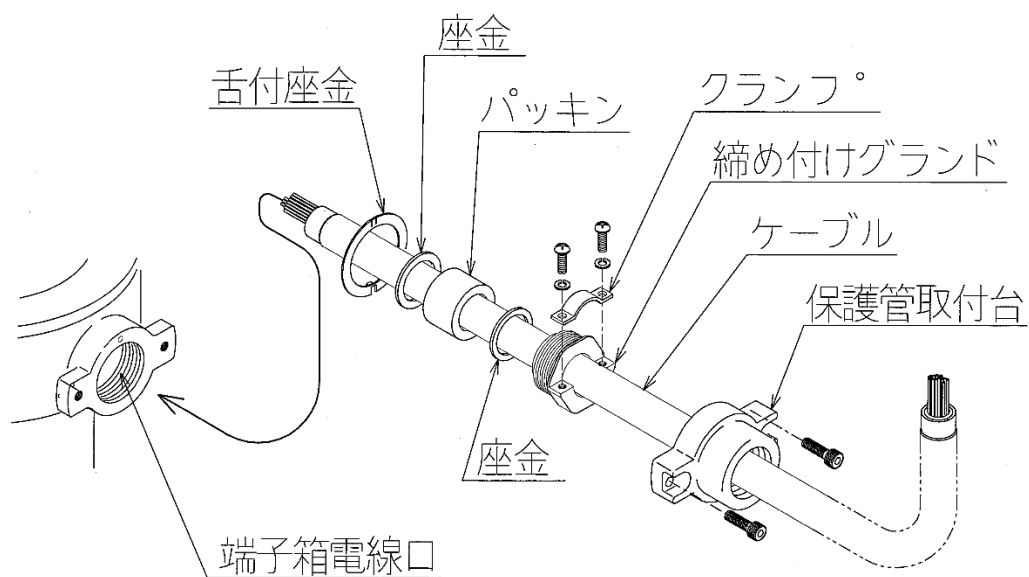
図5：耐圧パッキン式電線口詳細
