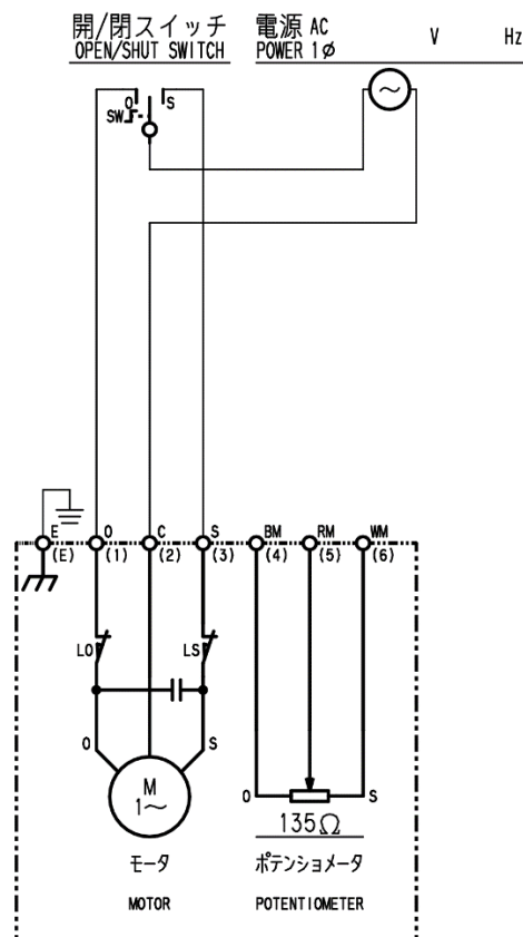
図 7 : C 形内部接続図
