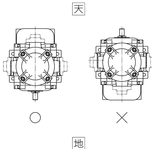
図1：据付け方向の制限
