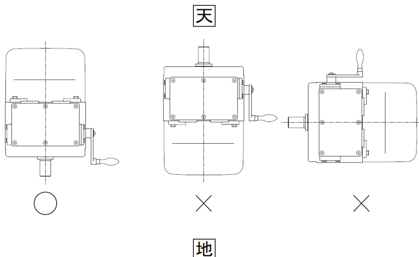
図 2：据付け方向の制限
