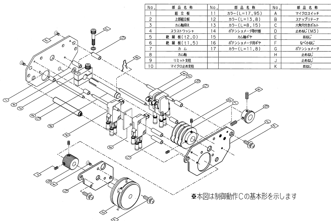
図 1 2 : スイッチ部の構造
