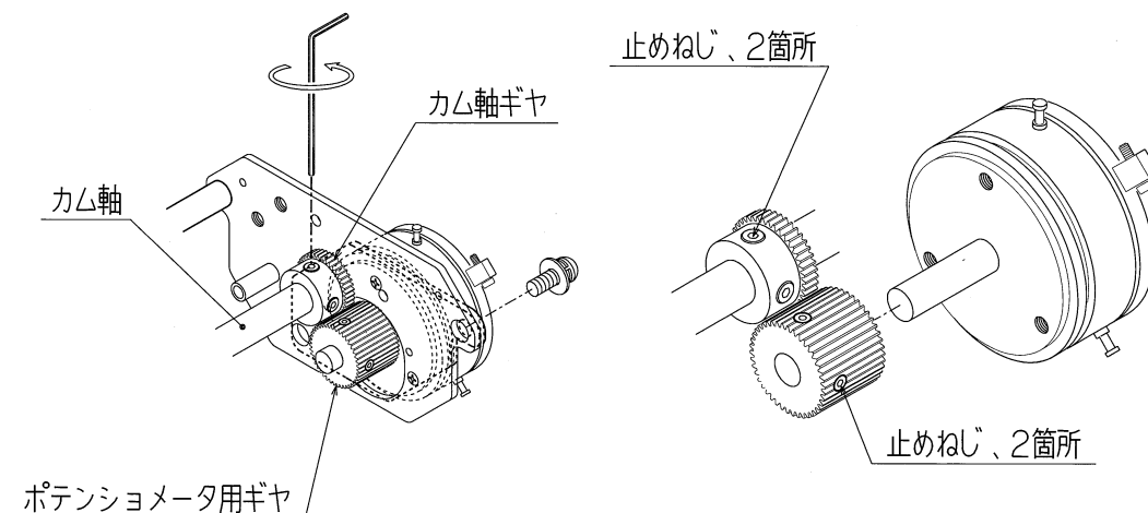
図 1 1 : ポテンシオメータの調整
