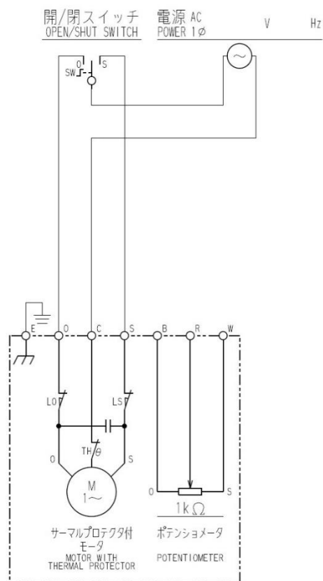
図 7 : C 形 (1kΩ) 内部接続図
