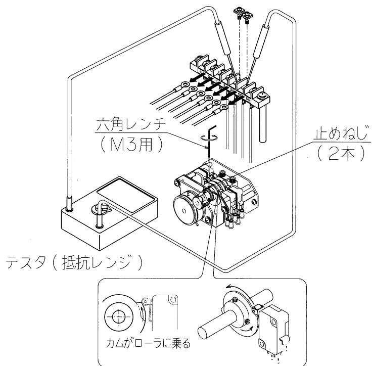
図9：スイッチ調整
