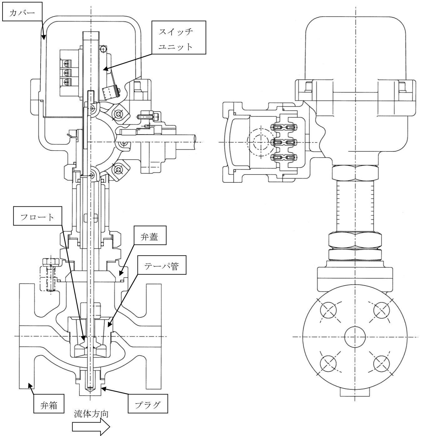
図3. dsAQ-243形 フローリレー構造図
