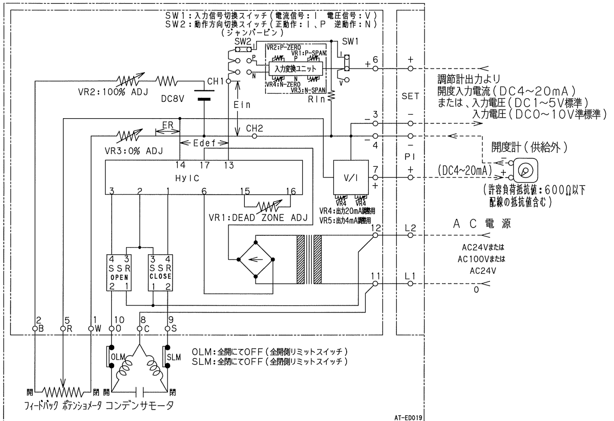
動作原理図
