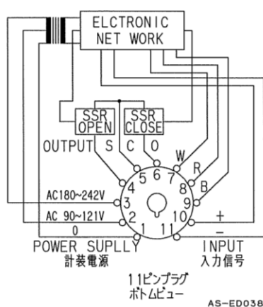
内部接続図
