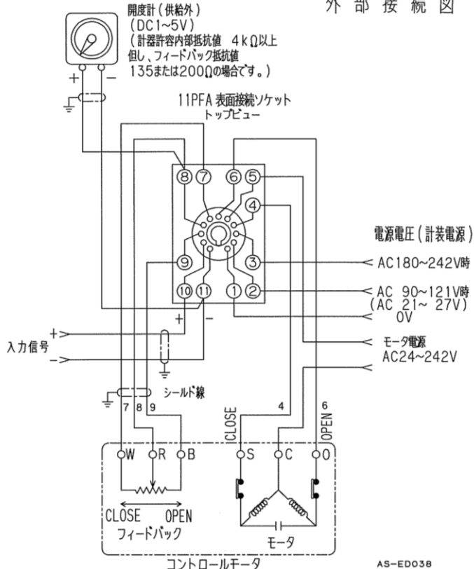
外部接続図
